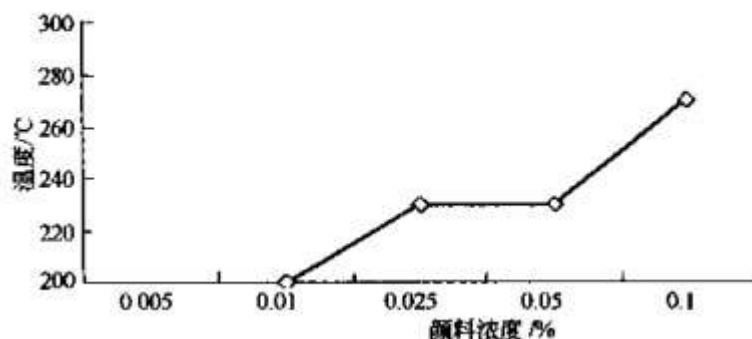
在 HDPE 中的耐温性
